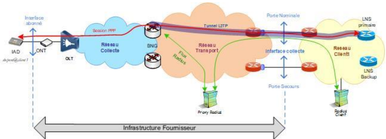
Figure 18 - Architecture collecte PPP livrée en L2TP
