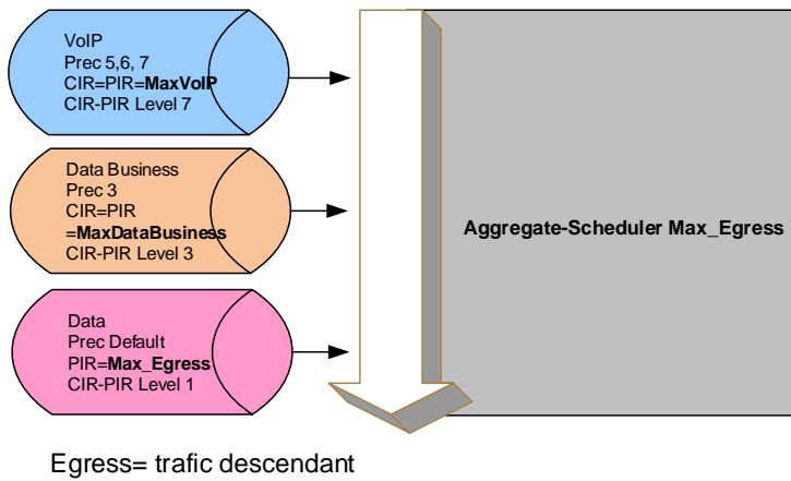
Figure 17 - Profil de QoS Abonné OPERA Office 100M en mode IPoE
