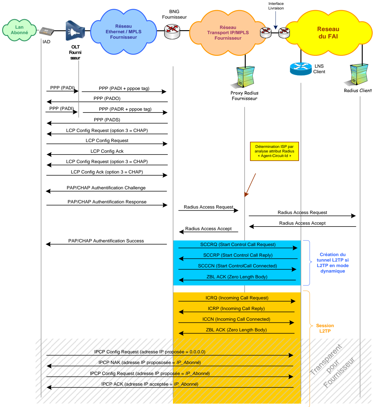
Figure 5 - Synthèse des échanges pour la création d'une session PPP-L2TP
