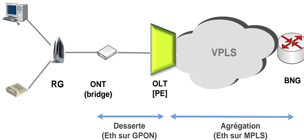
Figure 2 - Réseau de collecte GPON du service OPERA Office 100M
